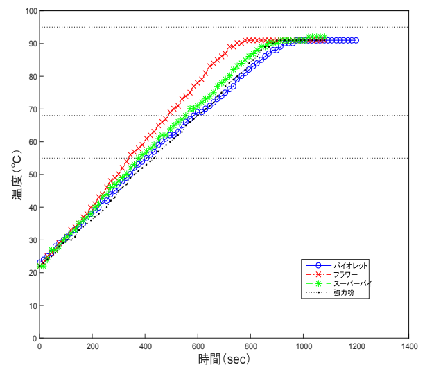
図7. (上)小麦粉水(小麦粉150g、水190g):バイオレット(印)とフラワー(×印)とスーパーバイオレット(*印)と強力粉ひまわり(・印)の電力値。(下)水温の時間変化。
