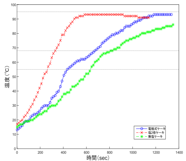
図 4. (上) 全卵をホイップした泡状生地の基本電極式ケーキ ( 印: 全卵 100g、小麦粉 50g、塩 0.6g、ふくらし粉 1.0g) と塩 2 倍電極式ケーキ ( × 印: 全卵 120g、小麦粉 60g、塩 1.2g、ふくらし粉 2.0g) と無塩電極式ケーキ ( * 印: 全卵 100g、小麦粉 50g、塩 0.0g、ふくらし粉 1.5g) の電力値。(下) 水温の時間変化。
